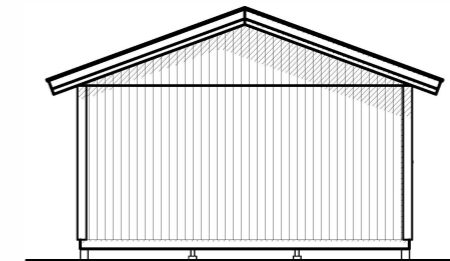
FASAD MOT
