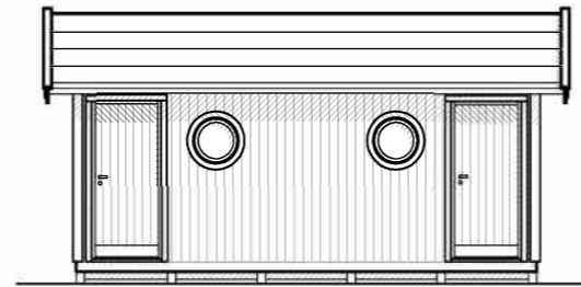
FASAD MOT
