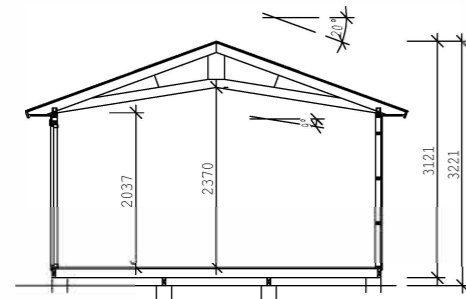
SEKTION
